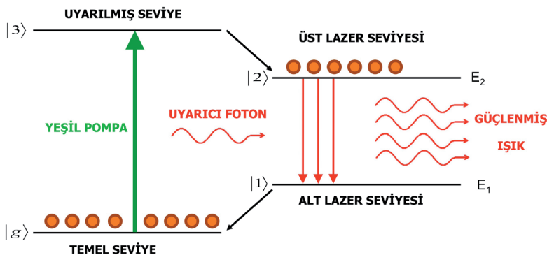
Şekil 4: Dört enerji düzeyi olan bir atomik sistemde, uyarılı ışımaya optik kazanç
