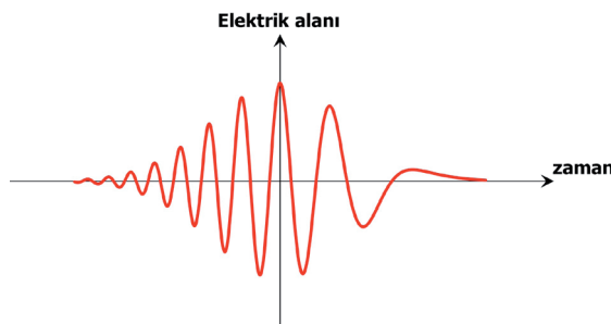
Şekil 8: Dağılımı değeri eksi olan bir ortamda ilerlerken değişime uğrayan optik darbenin elektrik alan dağılımı
