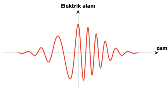
Şekil 7: Kerr ortamında ilerlerken, kendi başına faz kiplemesi sonucunda değişime uğrayan optik darbenin elektrik alan dağılımı
